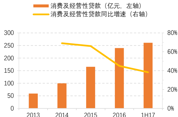
图 15：消费及经营性贷款增长有所放缓
